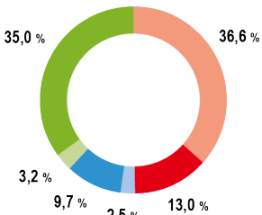
Energiemix Deutschland
