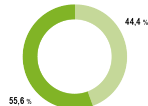
Energiemix Wasserkraft
