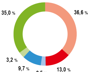
Energiemix Deutschland
