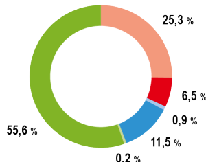
Verbleibender Energiemix
